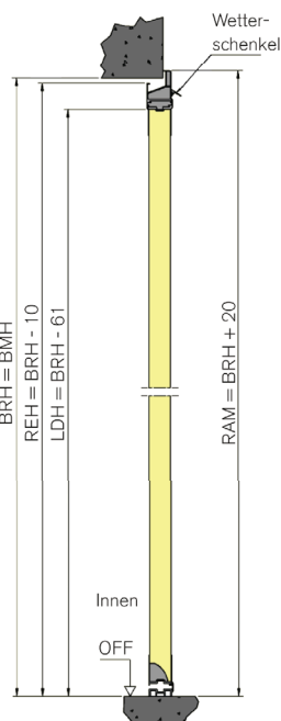
Nebentür mit Eckzarge
