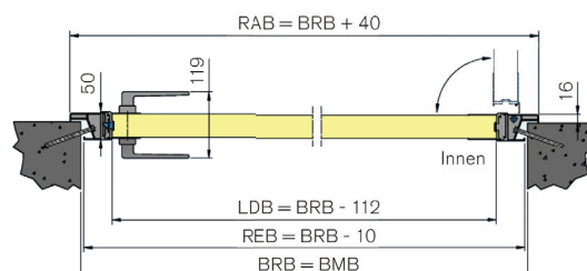
Nebentür mit Eckzarge
