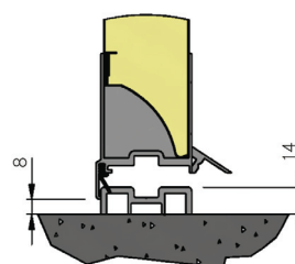
Detailsicht Schwelle (Vertikalschnitt)
