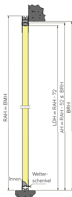
Nebentür mit Blockzarge hinter der Laibung
