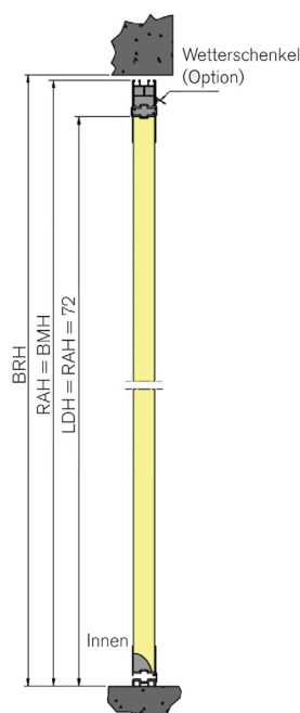
Nebentür mit Blockzarge zwischen der Laibung
