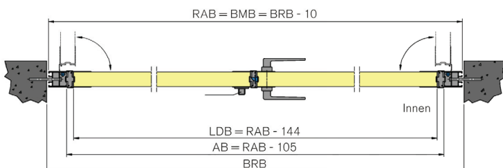
2-flügelige Nebentür mit Blockzarge zwischen der Laibung
