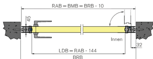
Nebentür mit Blockzarge zwischen der Laibung
