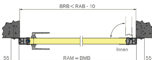
Nebentür mit Blockzarge hinter der Laibung (Hilfswinkel)
